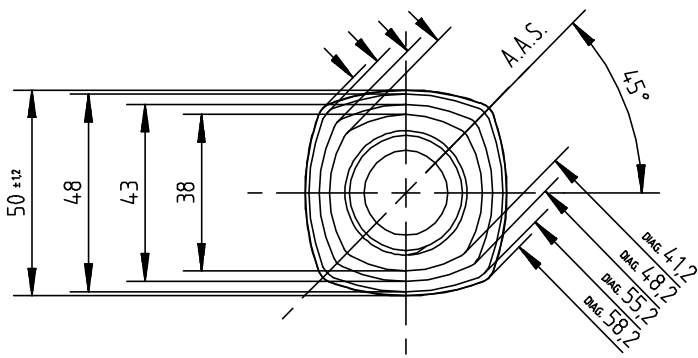
VISTA DALL'ALTO
