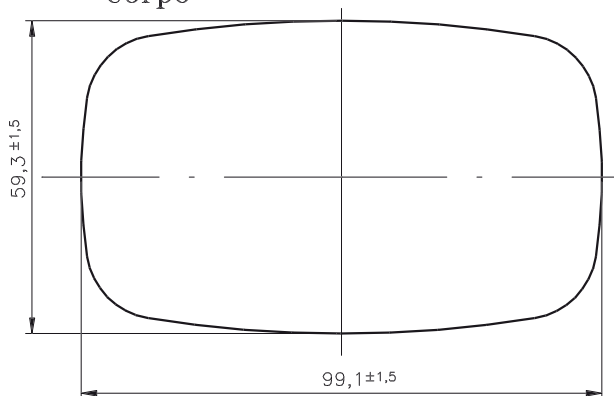
Sez.A-A Corpo
