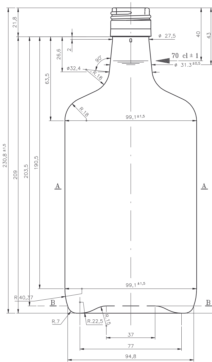
Sez.A-A Corpo
